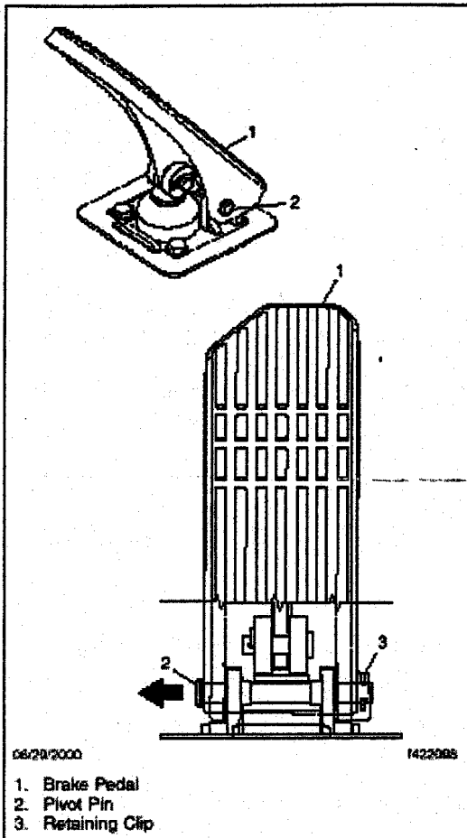
Fig. 1. Brake Pedal
